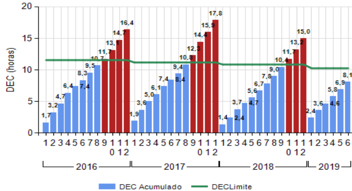
DEC – DURAÇÃO EQUIVALENTE DE INTERRUPÇÃO
