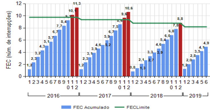
FEC - FREQUÊNCIA EQUIVALENTE DE INTERRUPÇÃO
